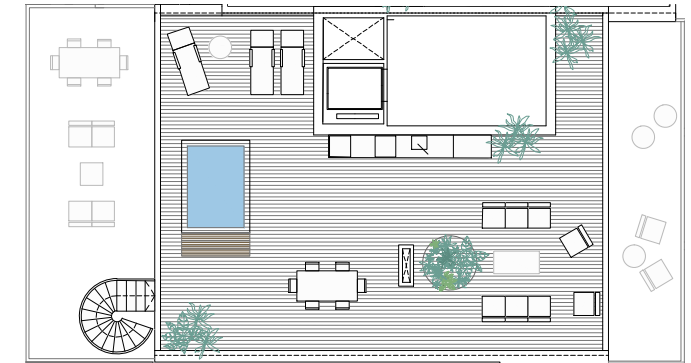
PLANTA SOLARIUM
