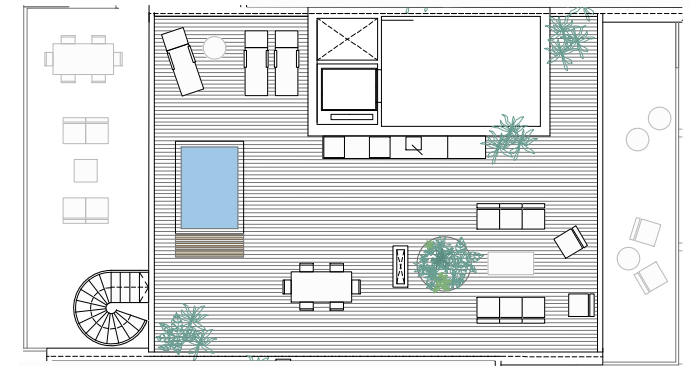
PLANTA SOLARIUM
